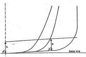
Figur 3 - Lasttankenes grænselinier jf. stk. 6
