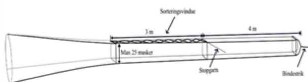
Figur 3. 4-panel fangstpose med et selektionspanel med diamantmasker på mindst 270 mm
