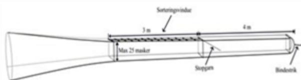
Figur 1. 4-panel fangstpose med et 180 mm kvadratmasket selektionspanel
