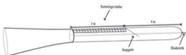
Figur 5. 2-panel fangstpose med et 180 mm kvadratmasket selektionspanel
